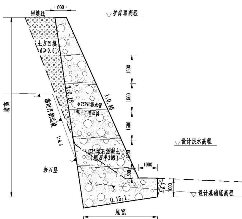
图 2-1 仰斜式挡土墙典型断面图(上游段)
