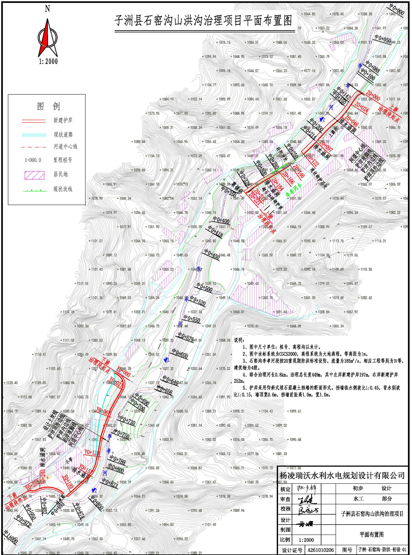
附图4 工程平面布置图
