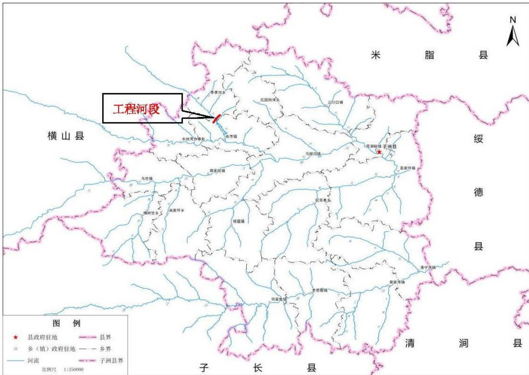
附图3 流域水系分布图
