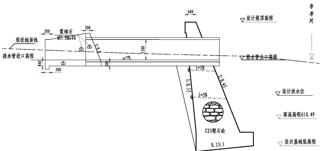
图 2-3 排水涵管典型断面设计图
