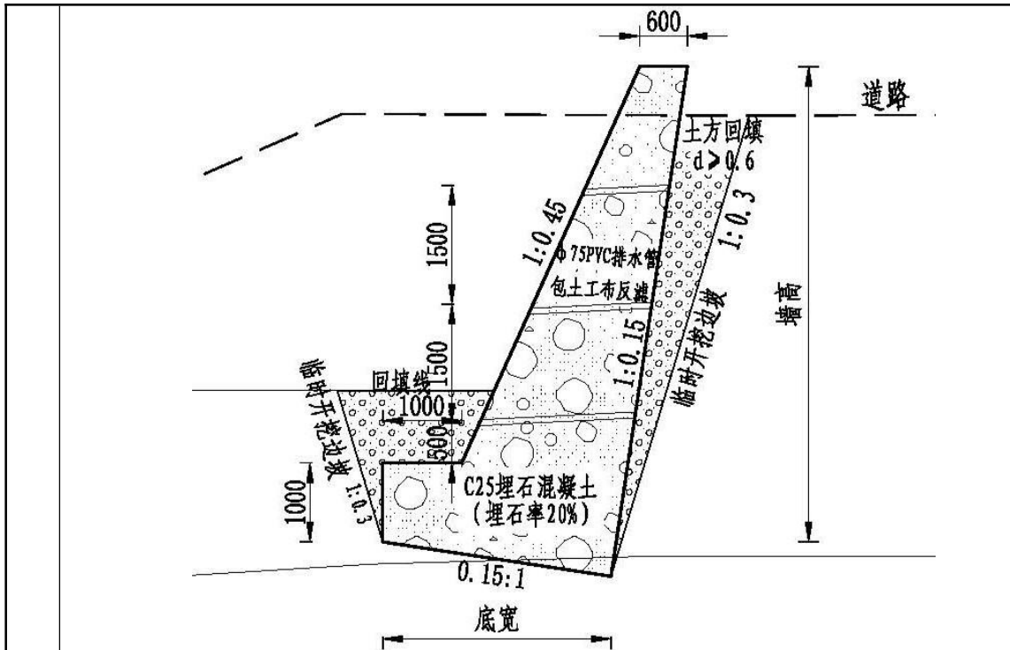
图 2-2 仰斜式挡土墙典型断面图（下游段）
