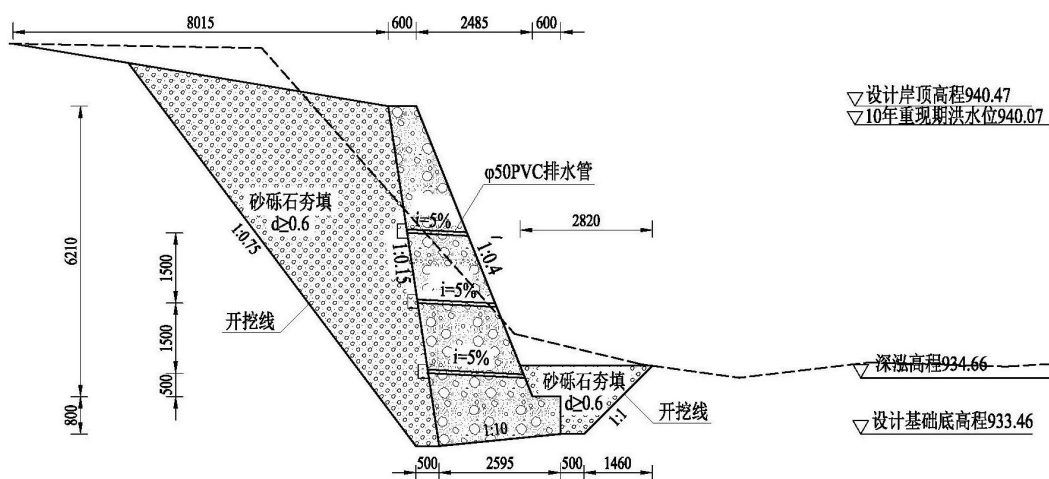
图 2-1 仰斜式挡土墙典型断面图
