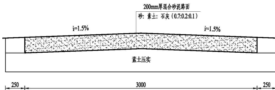
泥结石道路设计图
