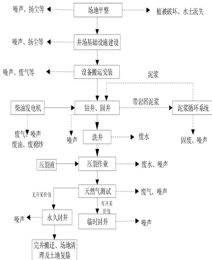
图2-6 项目主要工艺流程及产污环节
