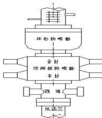
图 2-4 二开井口
