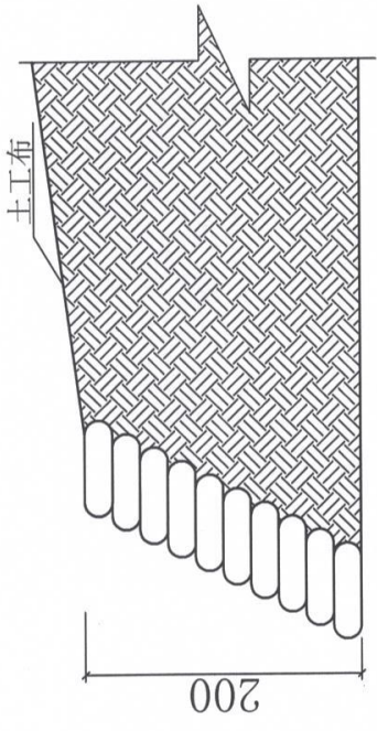
编织袋挡护断面图1:100
